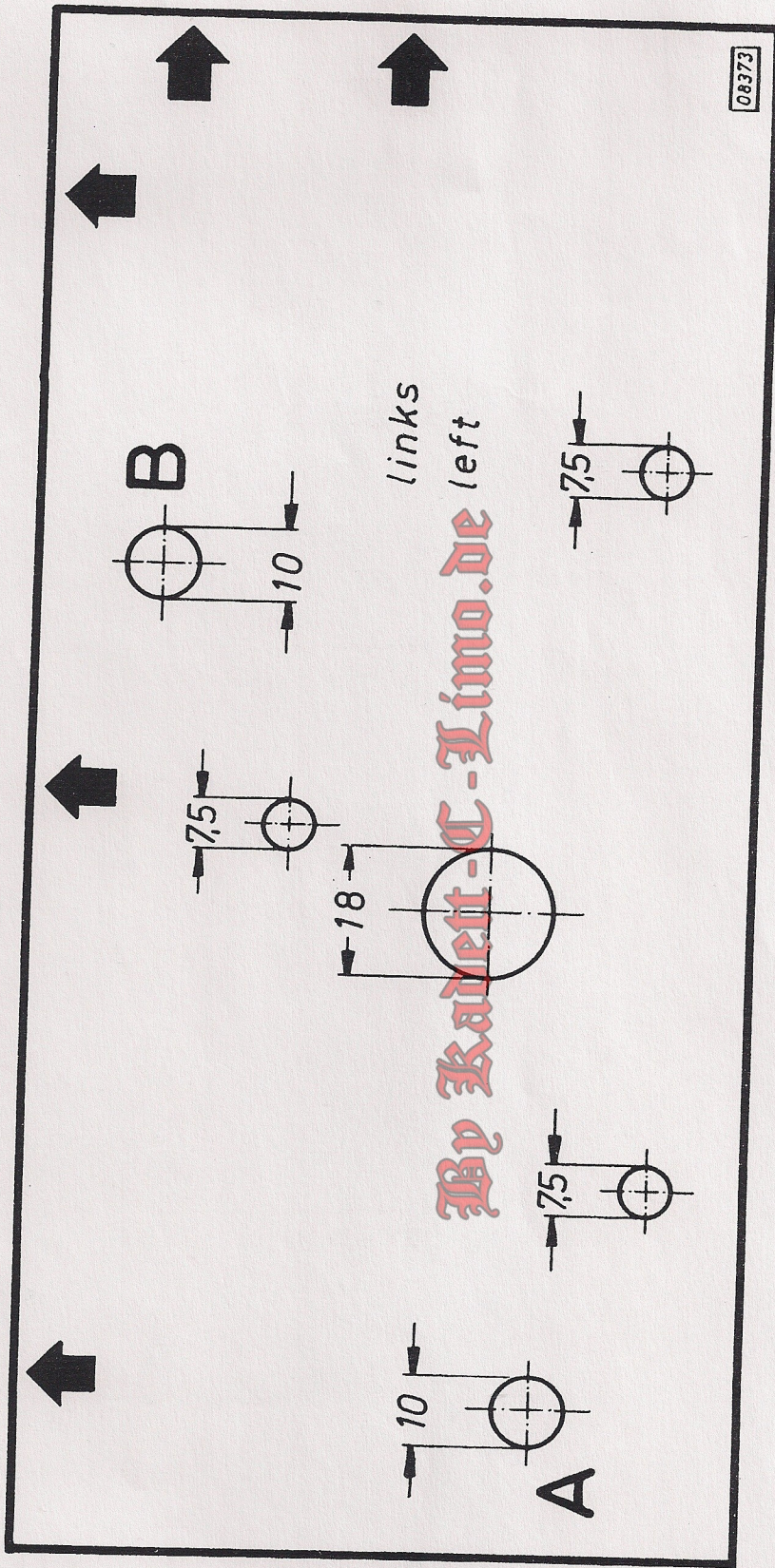
Bohrschablone für linken Scheinwerfer
